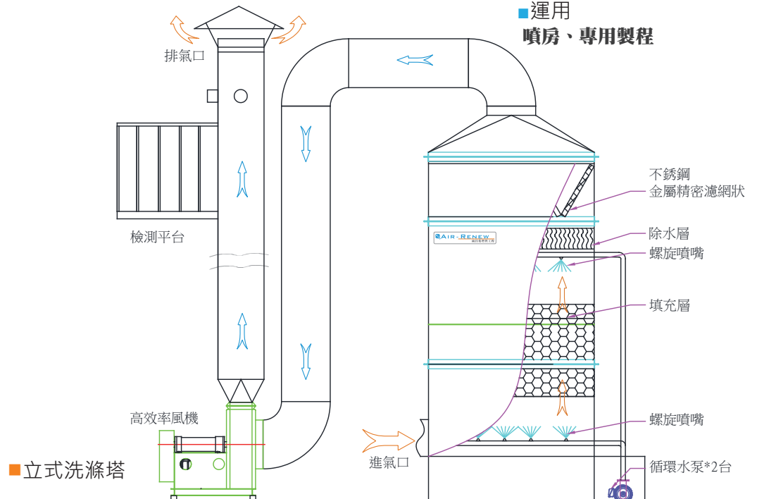
· 外觀示意圖
